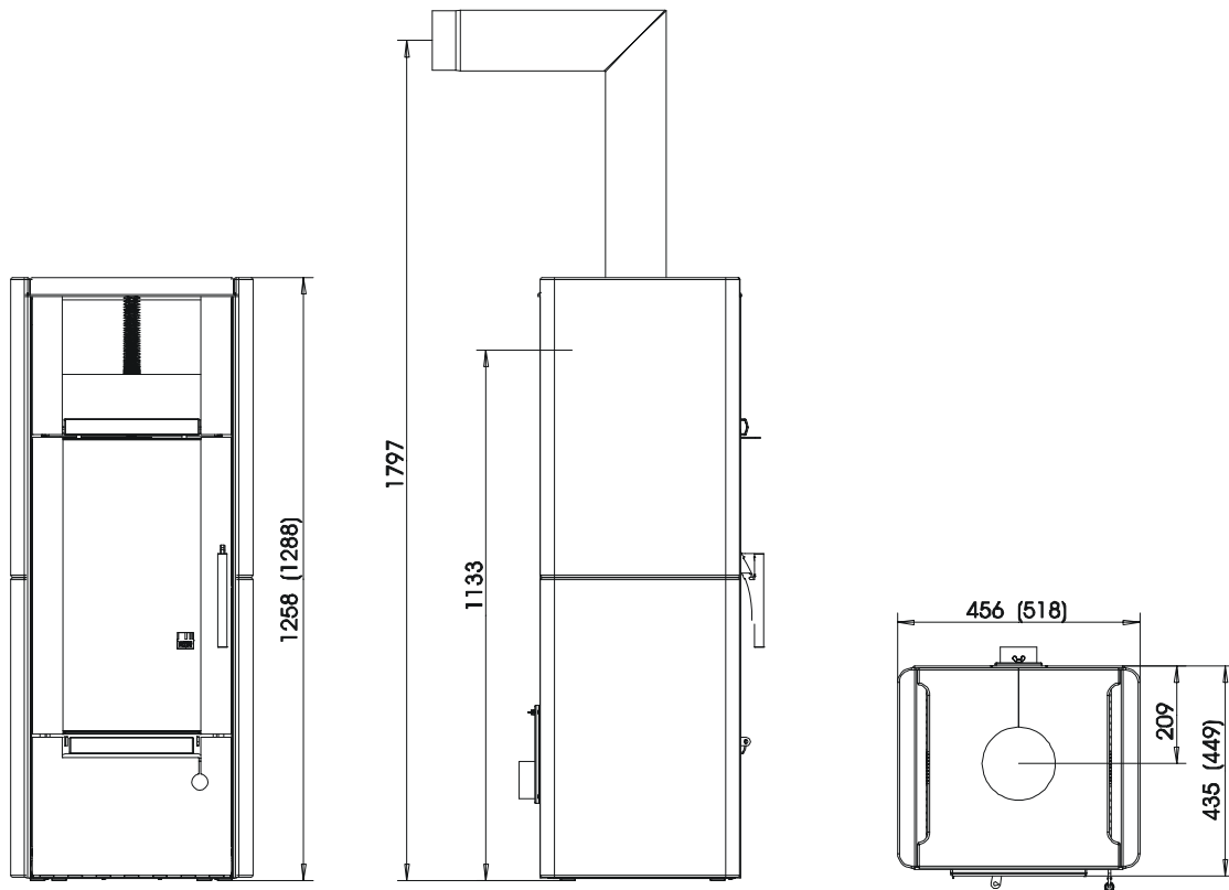
Fig. 1 ( )= Specksteinmaß
